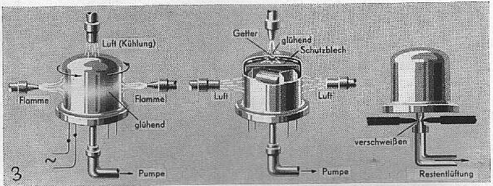
Bild 49. Verschweißen des Pumpröhrchens
