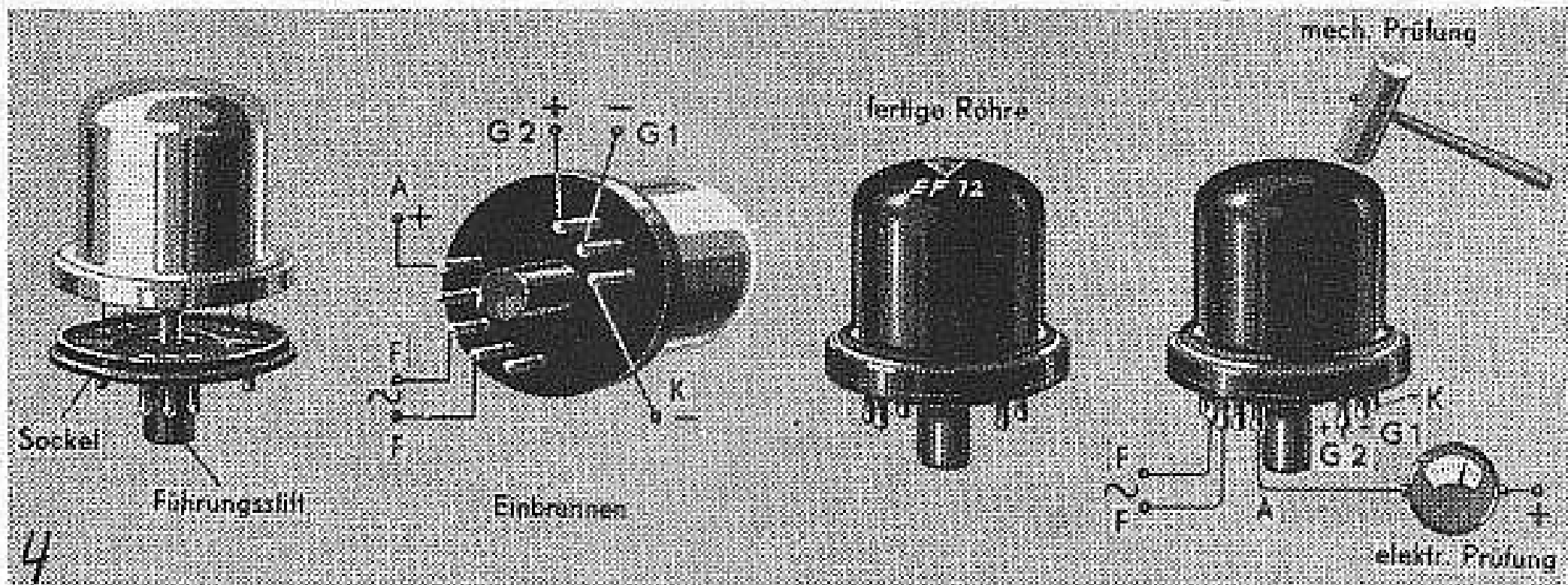
Bild 50. Anbringen des Bakelitsockels
