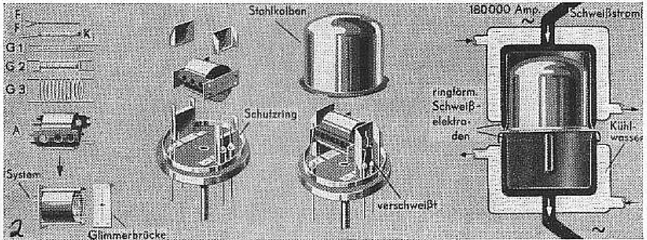
Bild 43. Zusammenbau des Systems aus den einzelnen Teilen
