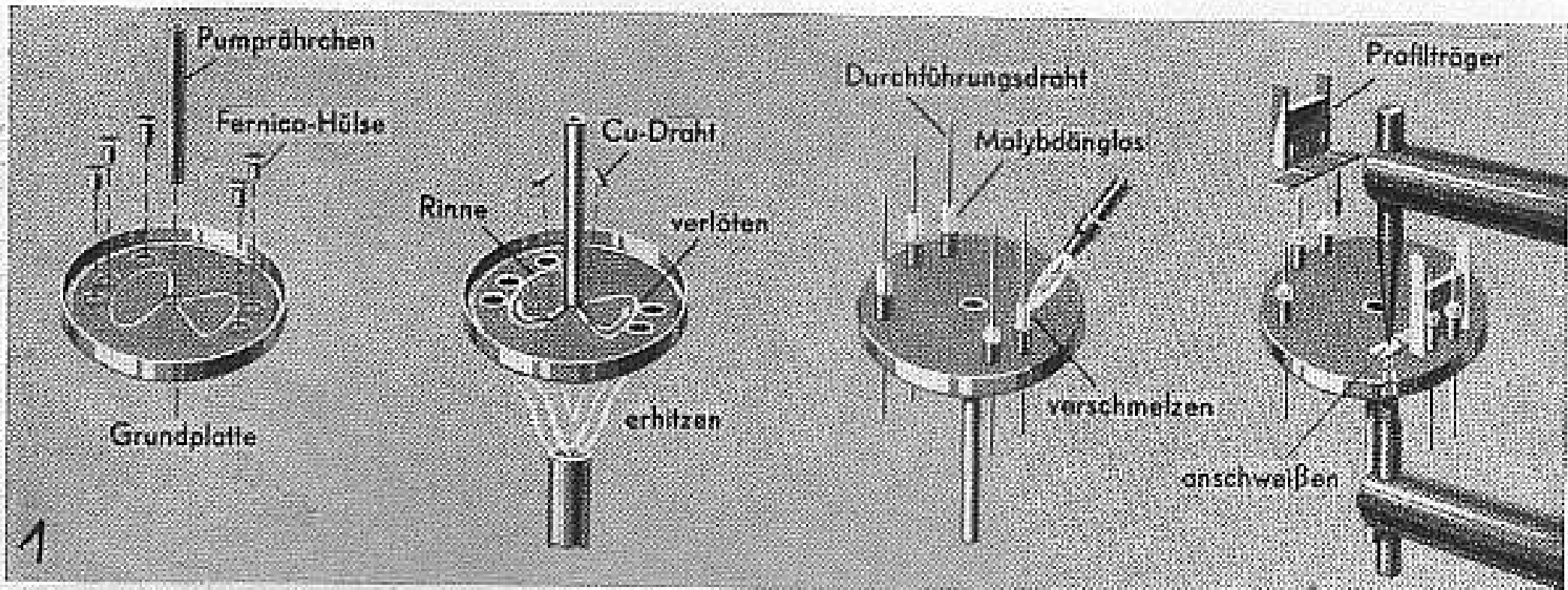
Bild 39. Grundplatte mit Durchführungen
